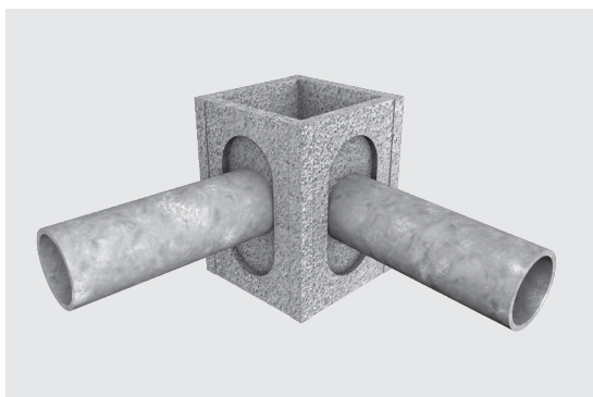
Esquema de entrada e saída de tubos em caixa dupla.
